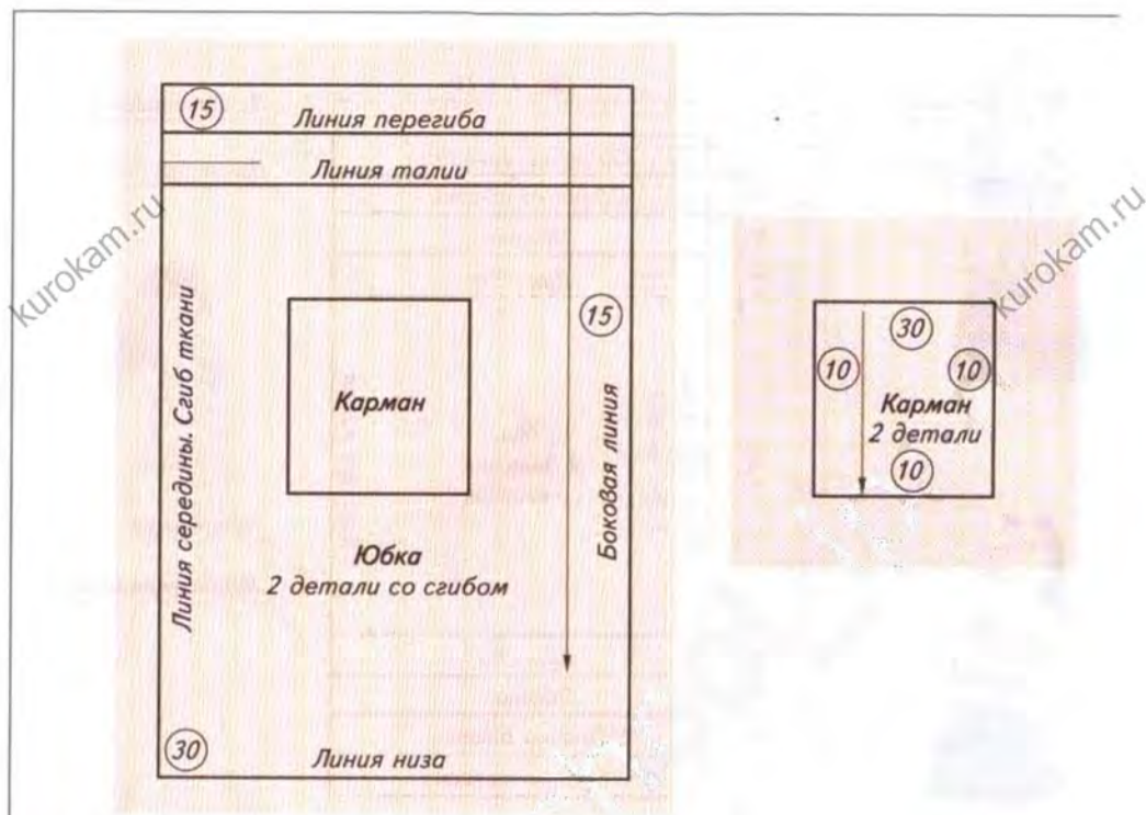
Рис. 56. Выкройка юбки с накладными карманами
