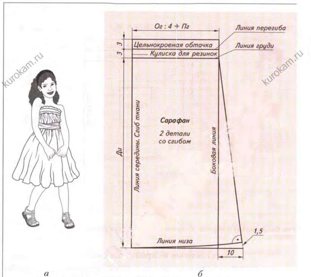
Рис. 54. Эскиз (а) и чертёж (б) сарафана с кулиской для резинок
