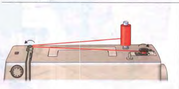
Рис. 71. Намотка нитки на шпульку
