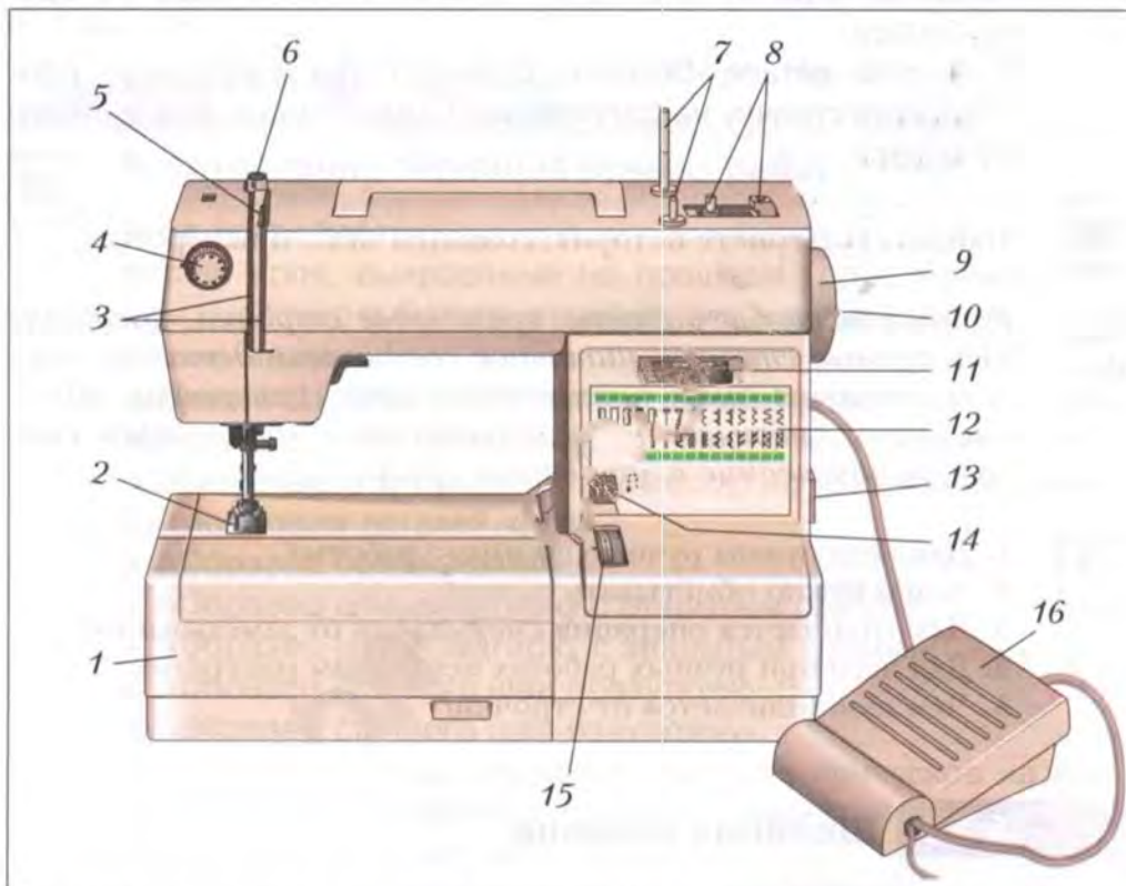
Рис. 69. Основные узлы швейной машины с электрическим приводом: 1 – платформа машины; 2 – лапка; 3 – прорези для нитки; 4 – регулятор натяжения верхней нитки; 5 – нитепритягиватель; 6 – устройство для натяжения нитки; 7 – штыри для катушек; 8 – моталка; 9 – маховик; 10 – стопорное кольцо; 11 – переключатель вида строчек; 12 – таблица выбора строчек; 13 – главный выключатель; 14 – клавиша шитья назад; 15 – регулятор длины стежка; 16 – педаль привода
