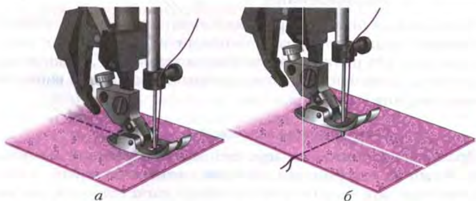
Рис. 75. Выполнение поворота строчки под углом: а – лапка и игла опущены; б – поворот ткани при поднятой лапке
