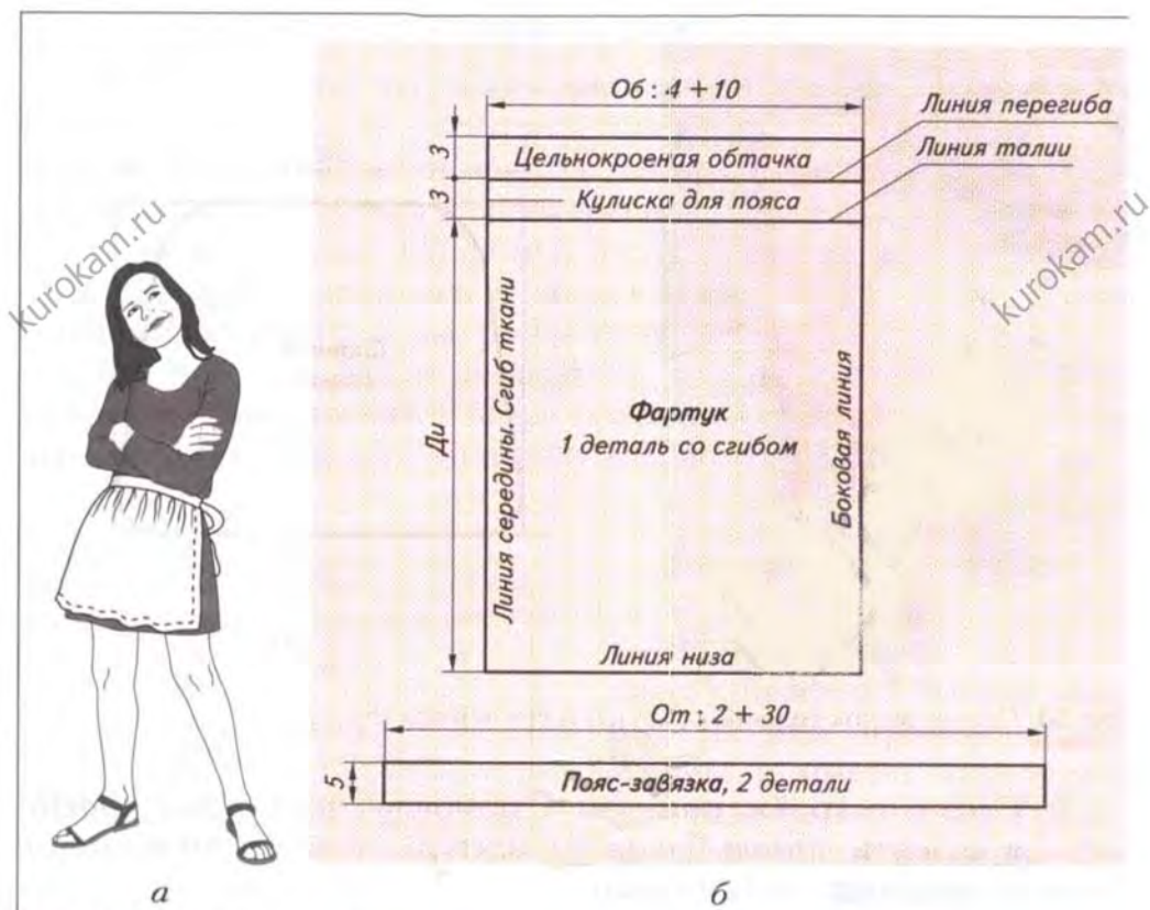
Рис. 52. Эскиз (а) и чертёж (б) фартука с поясом-кулиской и поясом-завязкой
