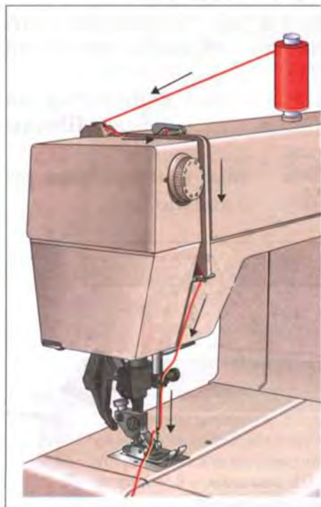
Рис. 72. Заправка верхней нитки
