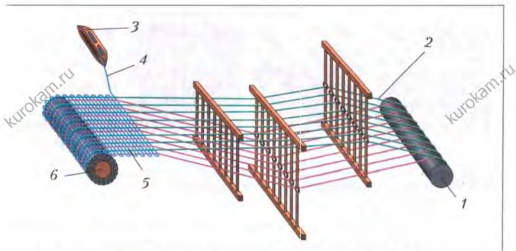
Рис. 42. Схема получения ткани на ткацком станке: 1 – навой; 2 – нити основы; 3 – челнок; 4 – нити утка; 5 – кромка; 6 – товарный валик
