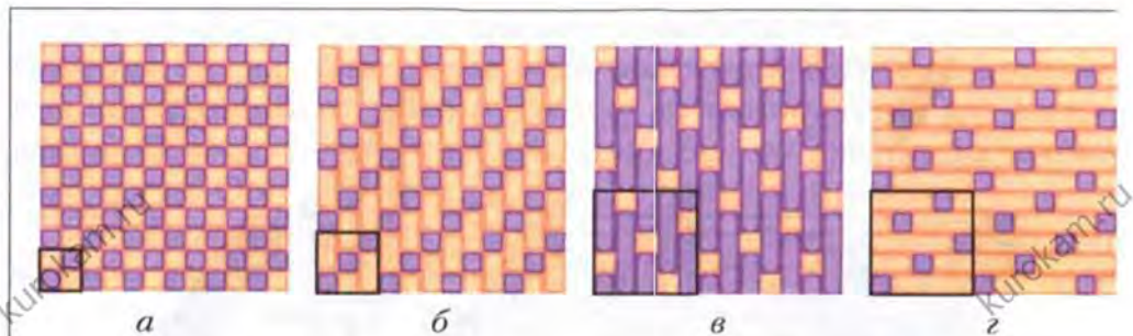
Рис. 43. Ткацкие переплетения: а – полотняное; б – саржевое; в – сатиновое; г – атласное. Выделенные участки – раппорт
