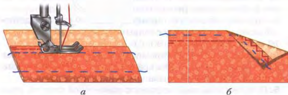
Рис. 80. Застрачивание: а – с закрытым срезом; б – с открытым срезом
