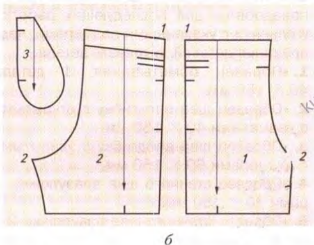
Рис. 57. Эскиз (а) и чертёж (б) бермудов из готовой выкройки
