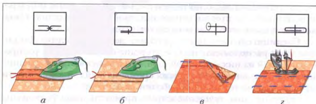
Рис. 85. Машинные швы и их условное обозначение: а – стачной вразутюжку; б – стачной взаутюжку; в – вподгибку с открытым обметанным срезом; г – вподгибку с закрытым срезом
