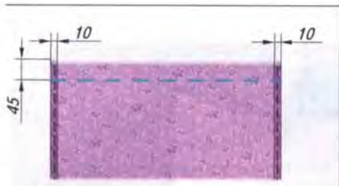
Рис. 87. Обработка боковых срезов фартука
