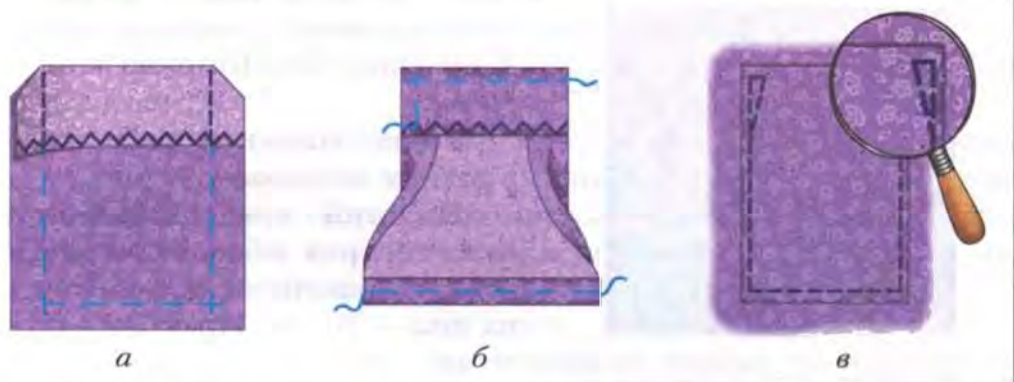
Рис. 92. Обработка накладного кармана: а – обработка верхнего среза; б – замётывание срезов; в – настрачивание кармана на изделие
